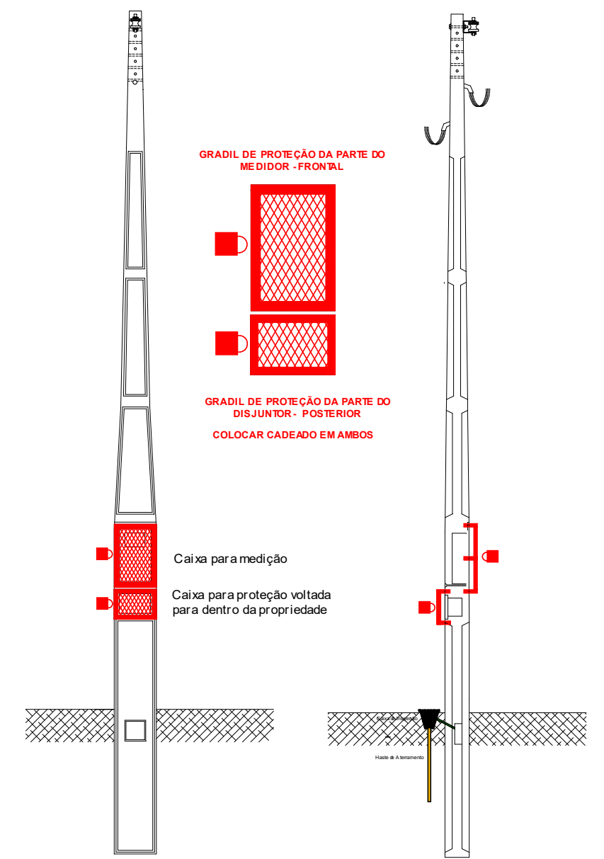
Padrão de Entrada com Caixa Incorporada – Instalação Voltado para Calçada
