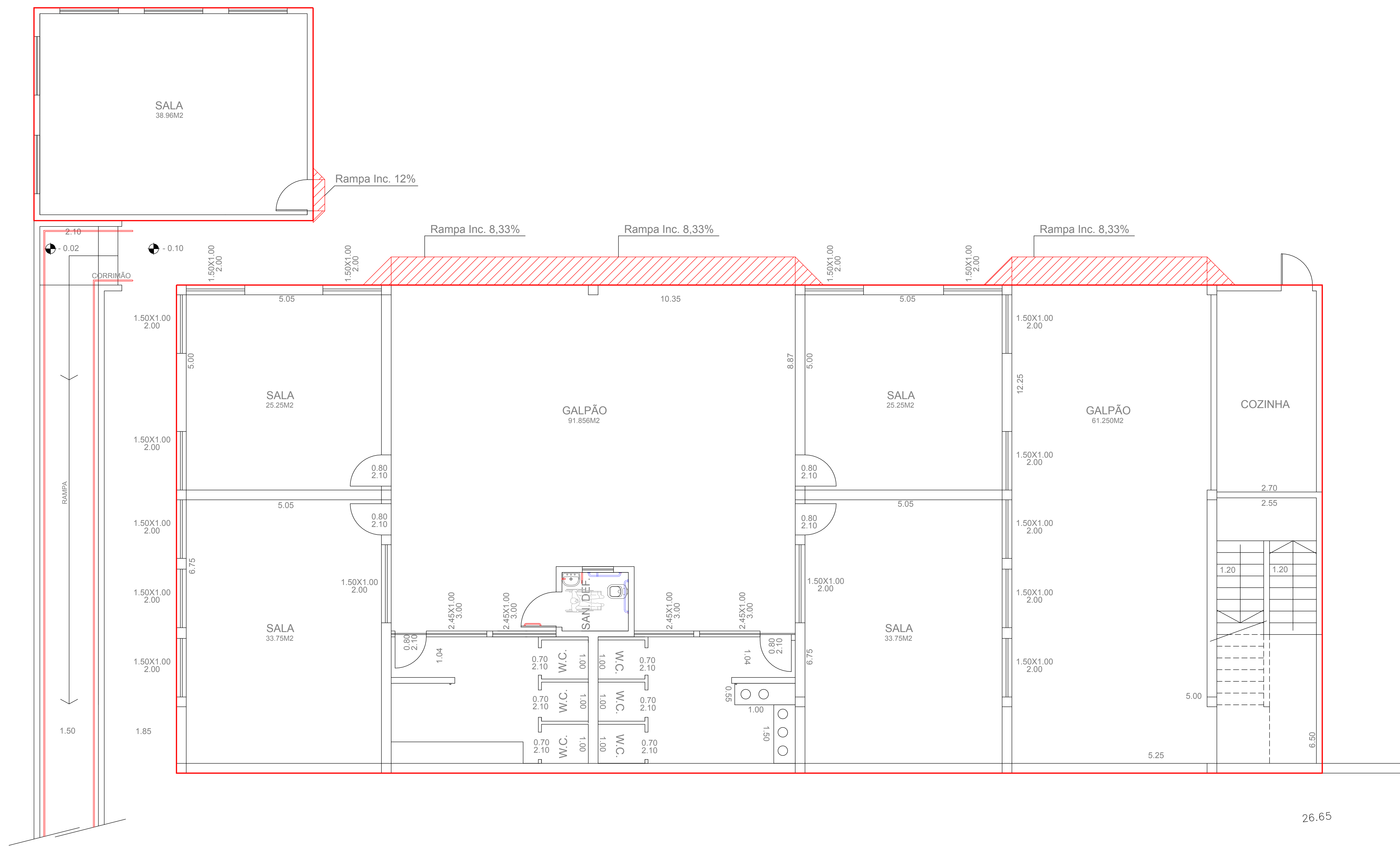
PLANTA PAV. INFERIOR
