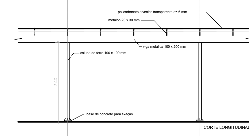
CORTE LONGITUDINAL DA COBERTURA ESC. 1.2
