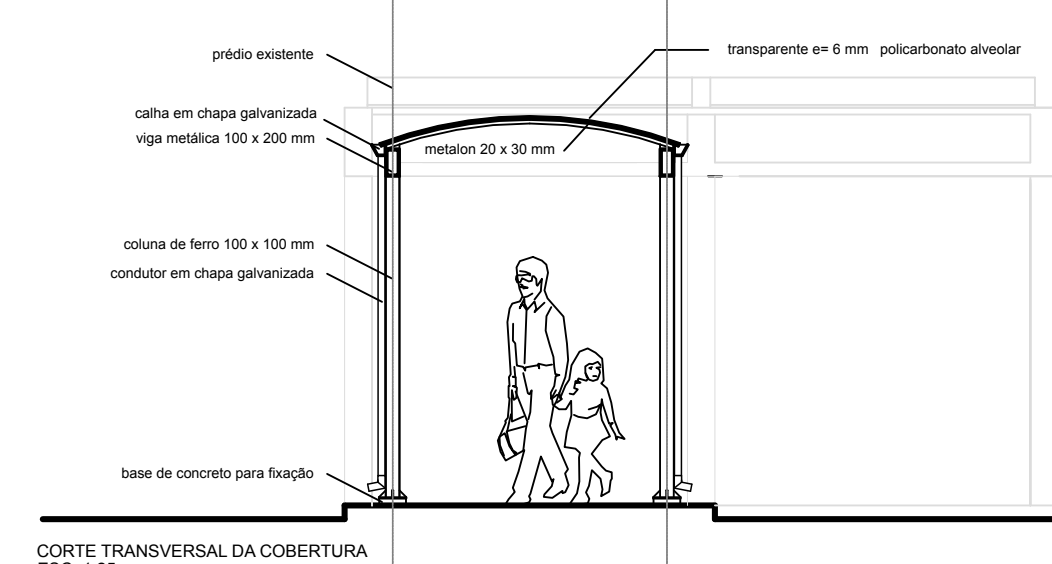
CORTE TRANSVERSAL DA COBERTURA ESC: 1:25
