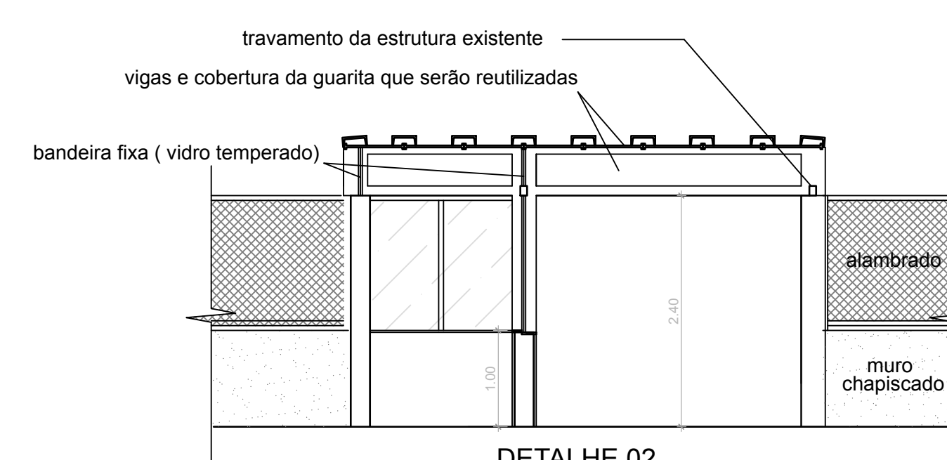
DETALHE 02 RELOCAÇÃO DA GUARITA ESCALA 1:50
