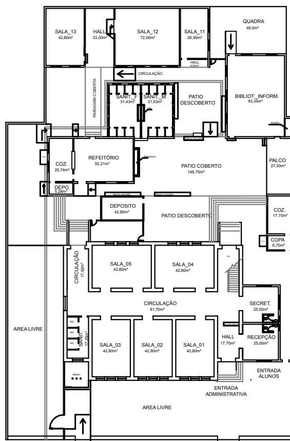
Planta_Pvto Térreo S/Escala
