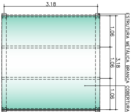
PLANTA DA PASSARELA
