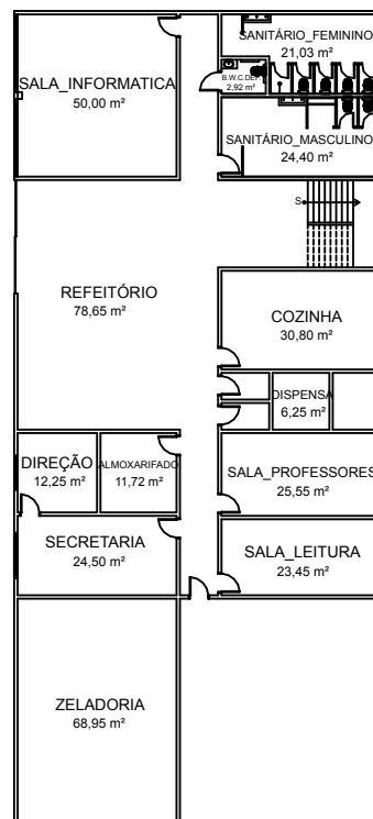
Planta Baixa S/Escala
