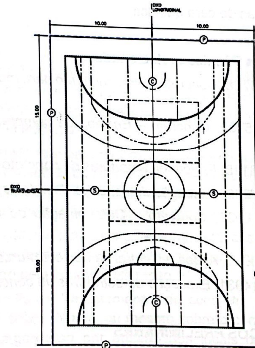
PAGINAÇÃO DA QUADRA DE CONCRETO ARMADO SEM ESCALA
