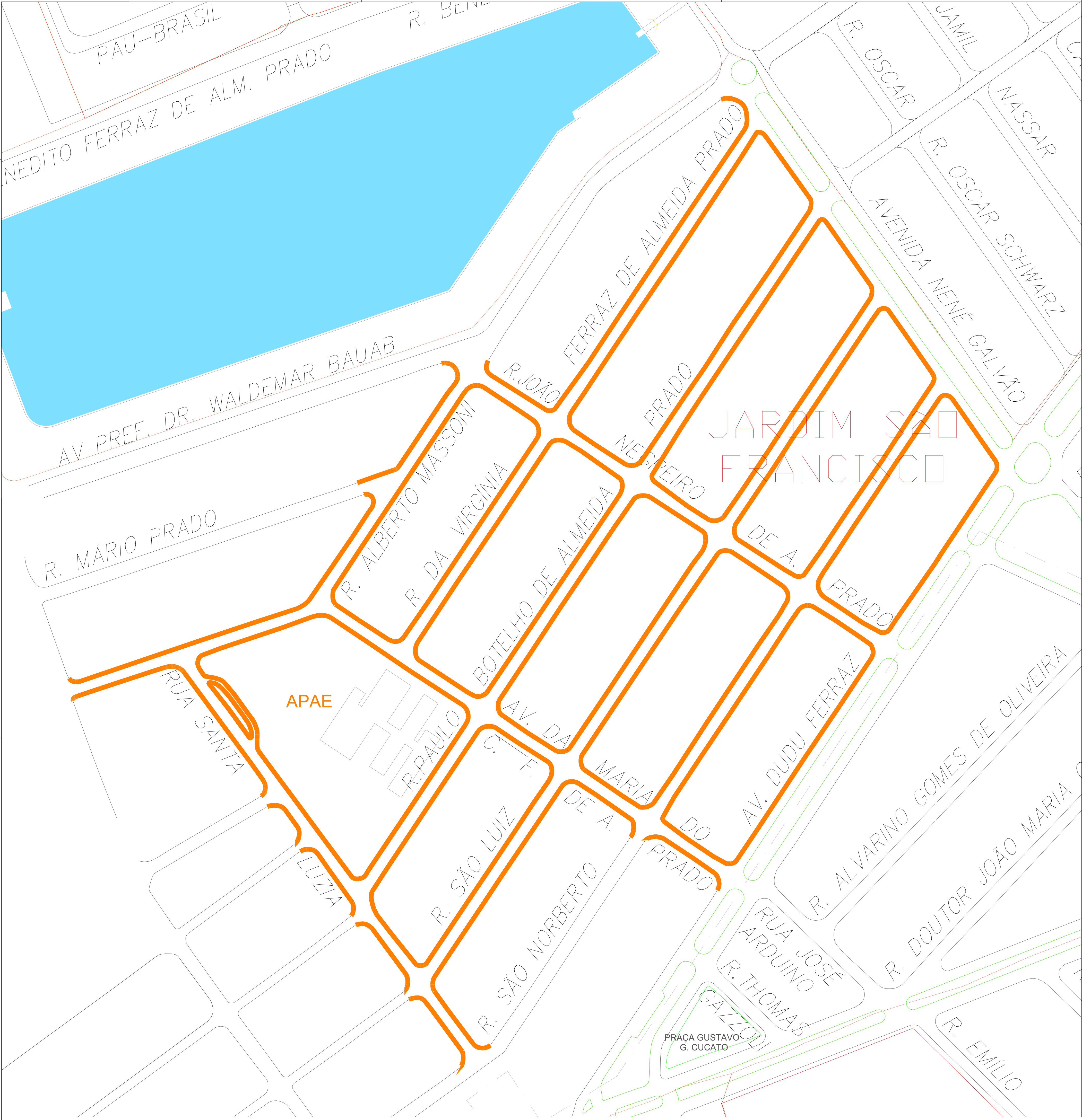
PLANTA DE LIMPEZA E TRATAMENTO DE GUIAS E SARJETAS ESCALA 1:1250
