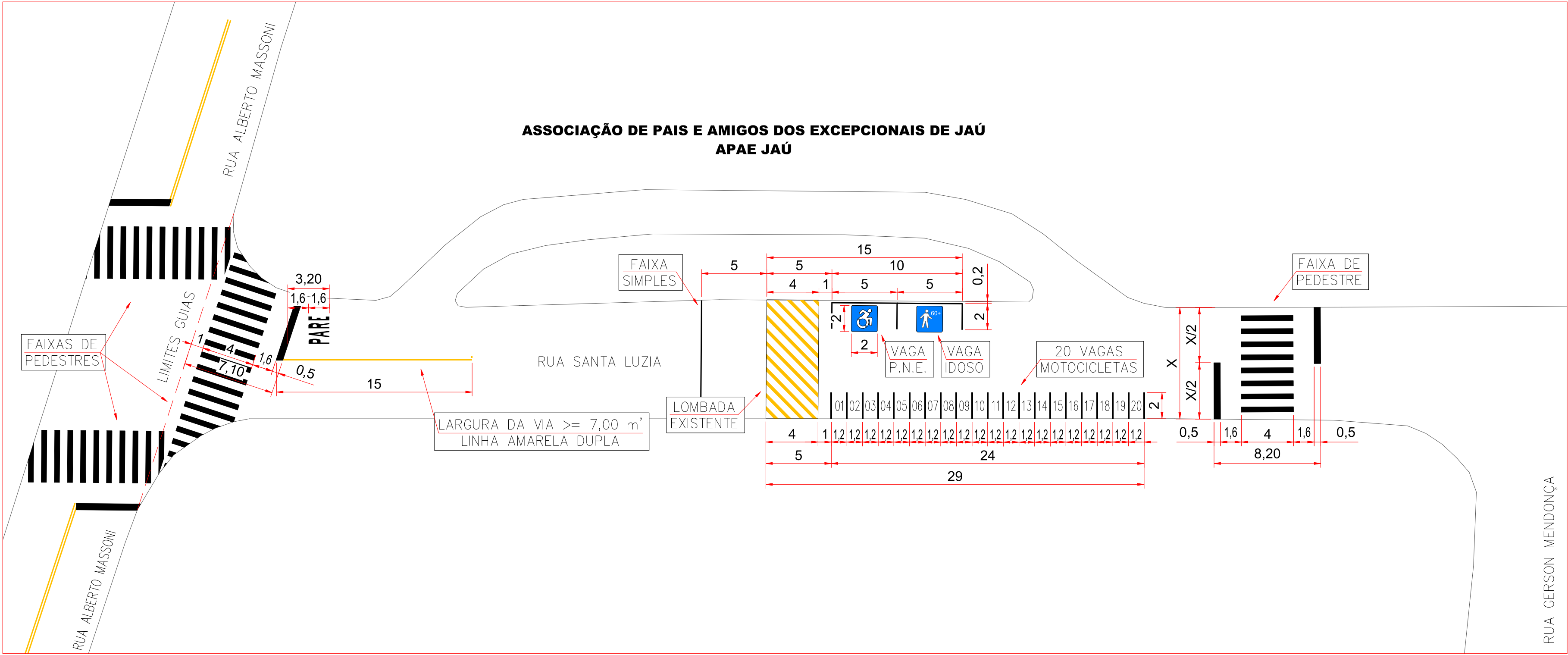
DETALHE A - SINALIZAÇÃO ESCALA 1:250
