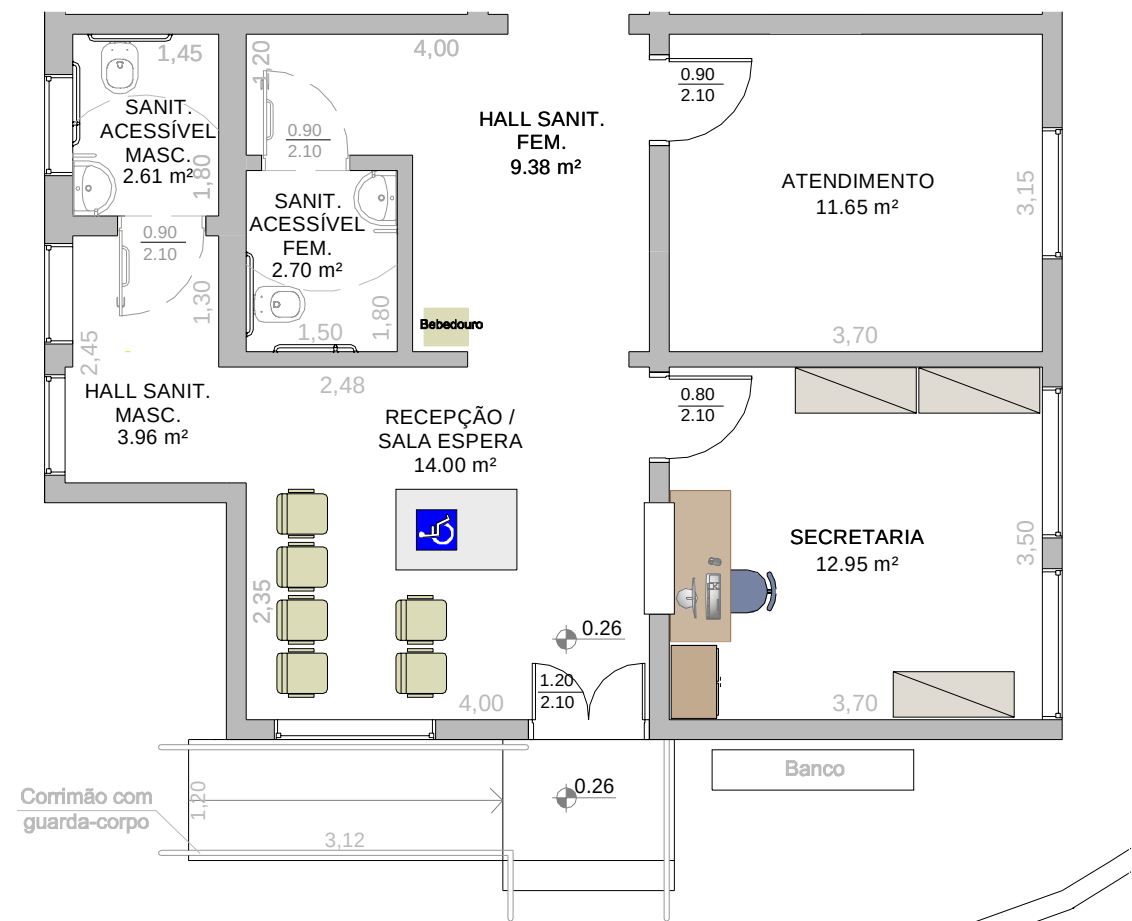
PLANTA LAYOUT - RECEPÇÃO ESCALA 1:100
