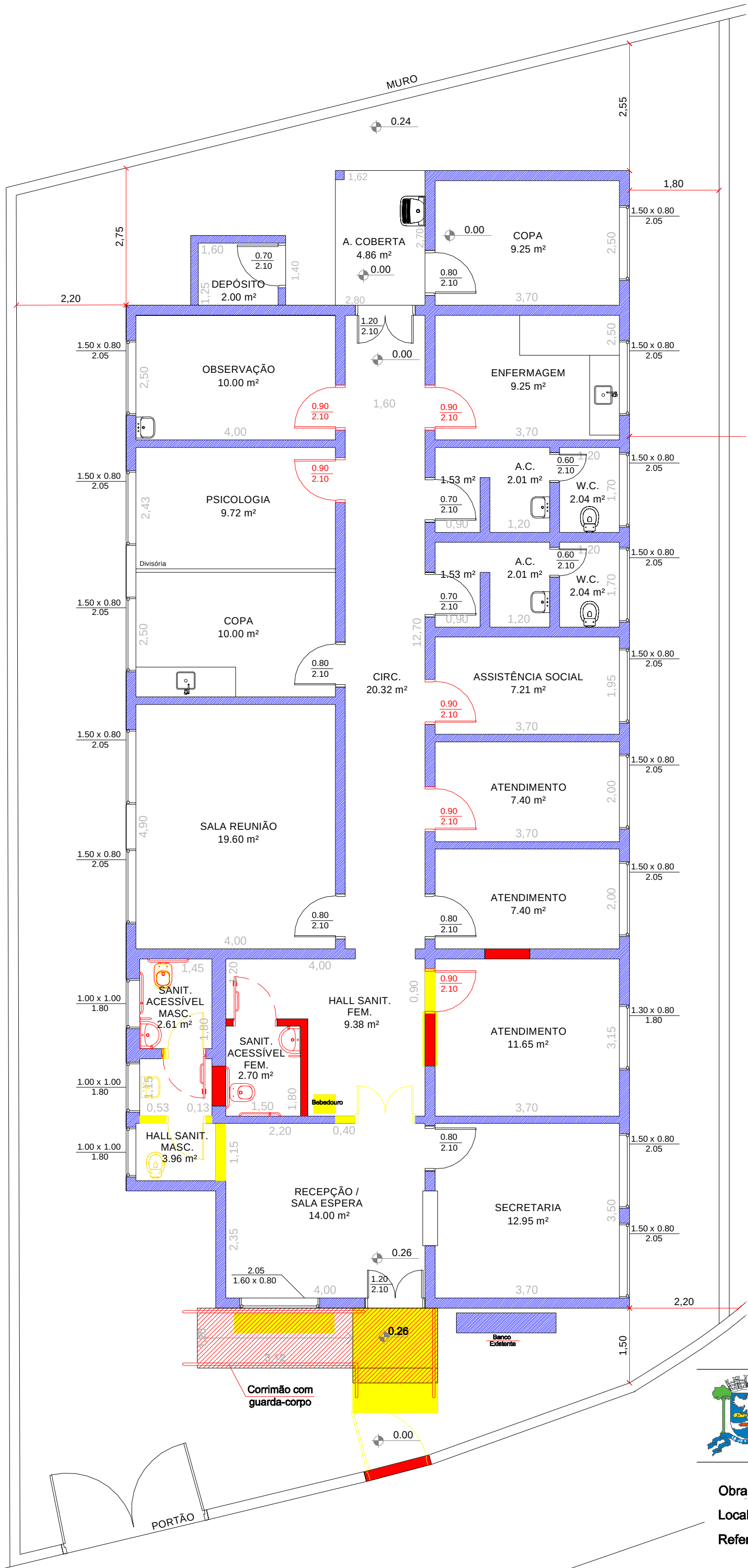
PLANTA DEMOLIR E CONSTRUIR ESCALA 1:100
