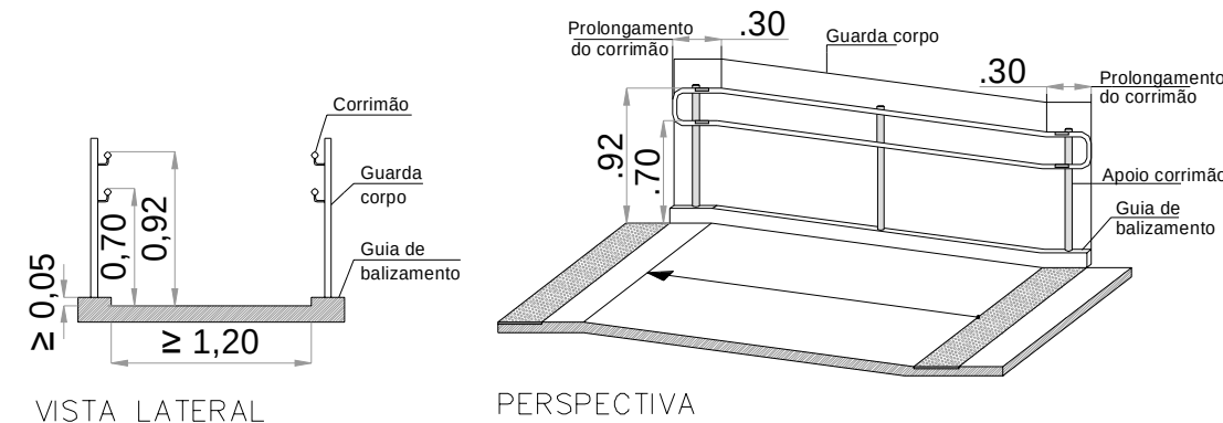
VISTA LATERAL
